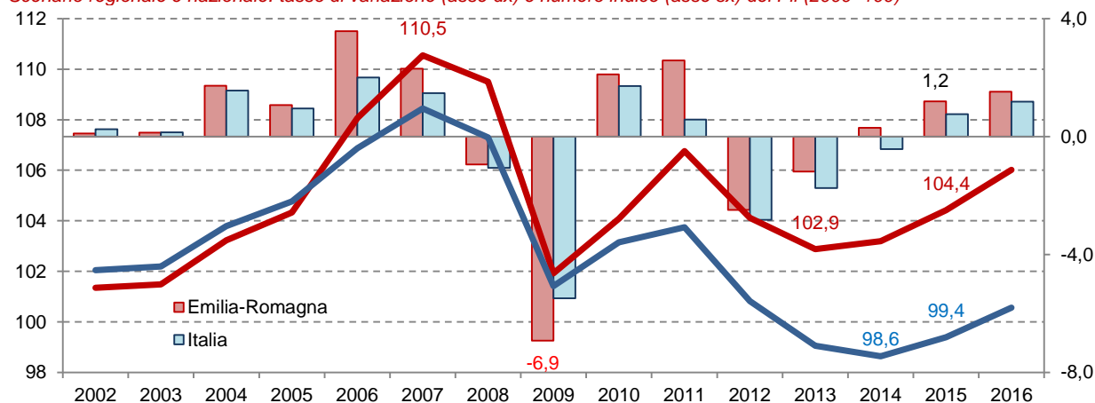
Scenario regionale e nazionale: tasso di variazione (asse dx) e numero indice (asse sx) del Pil (2000=100)
